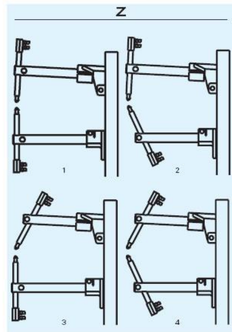
Grande flexibilité grâce aux différentes configurations de travail possibles
